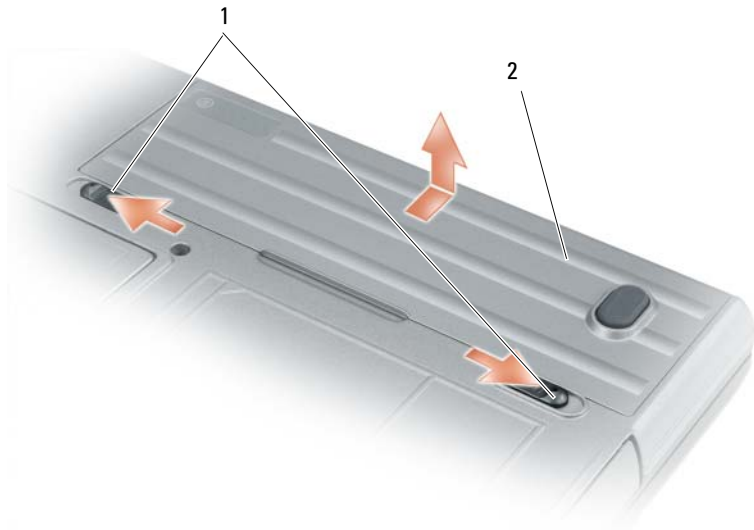
1 전지 베이 분리 래치 2 전지
