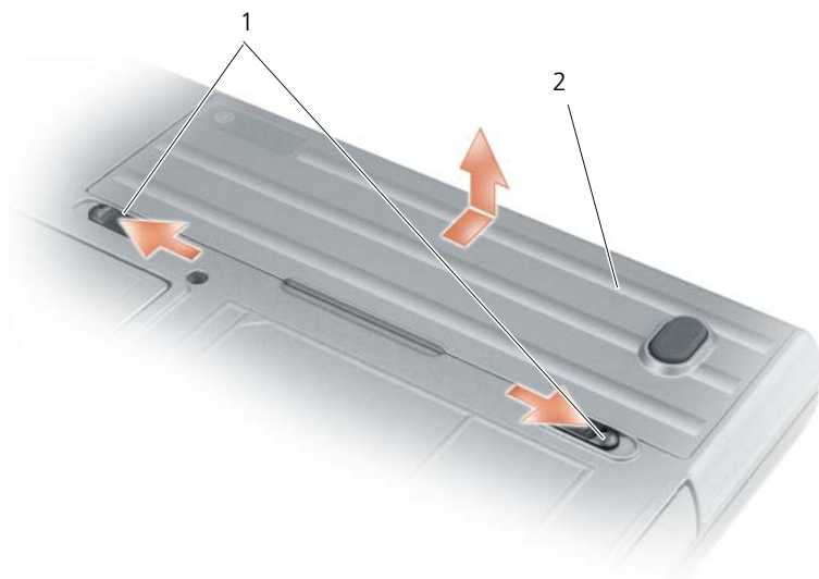
1 バッテリーベイリリース ラッチ 2 バッテリー ラッチ
